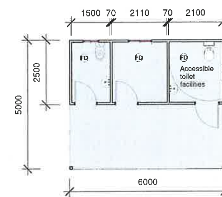
2 TOILETS 1 : 100
