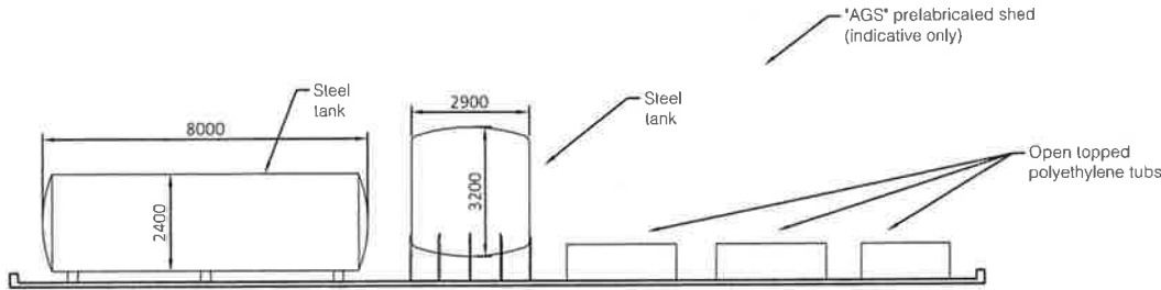
Section A-A (Scale A)
